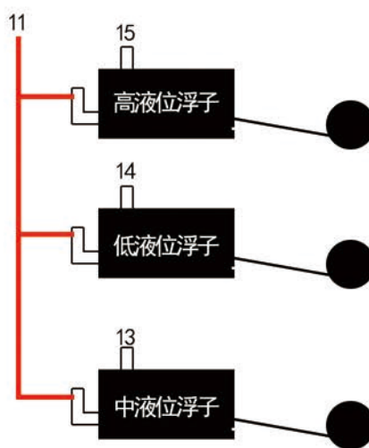
浮子型液位检测
